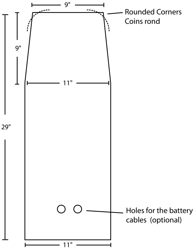
Back Of The Seat Dossier du siège
